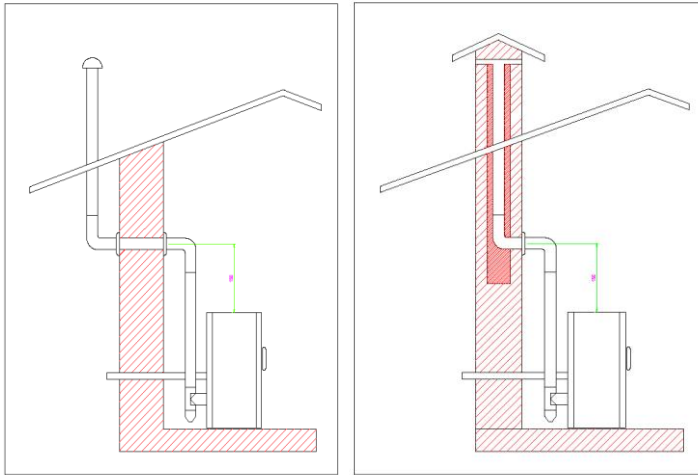
Σχήμα 1 - Τρόποι εγκατάστασης
