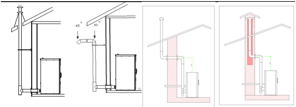
Εικόνα 4.2 Παραδείγματα εγκατάστασης καπνοδόχου
